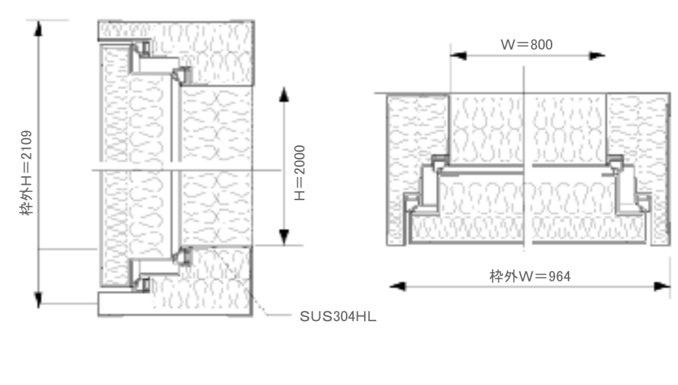
標準断面図
