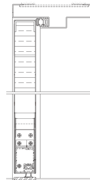
標準縦断面図
