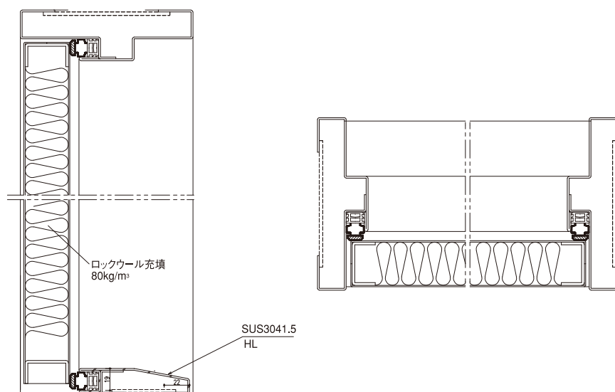
標準断面図
